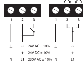
ЭЛЕКТРИЧЕСКОЕ ПОДКЛЮЧЕНИЕ
